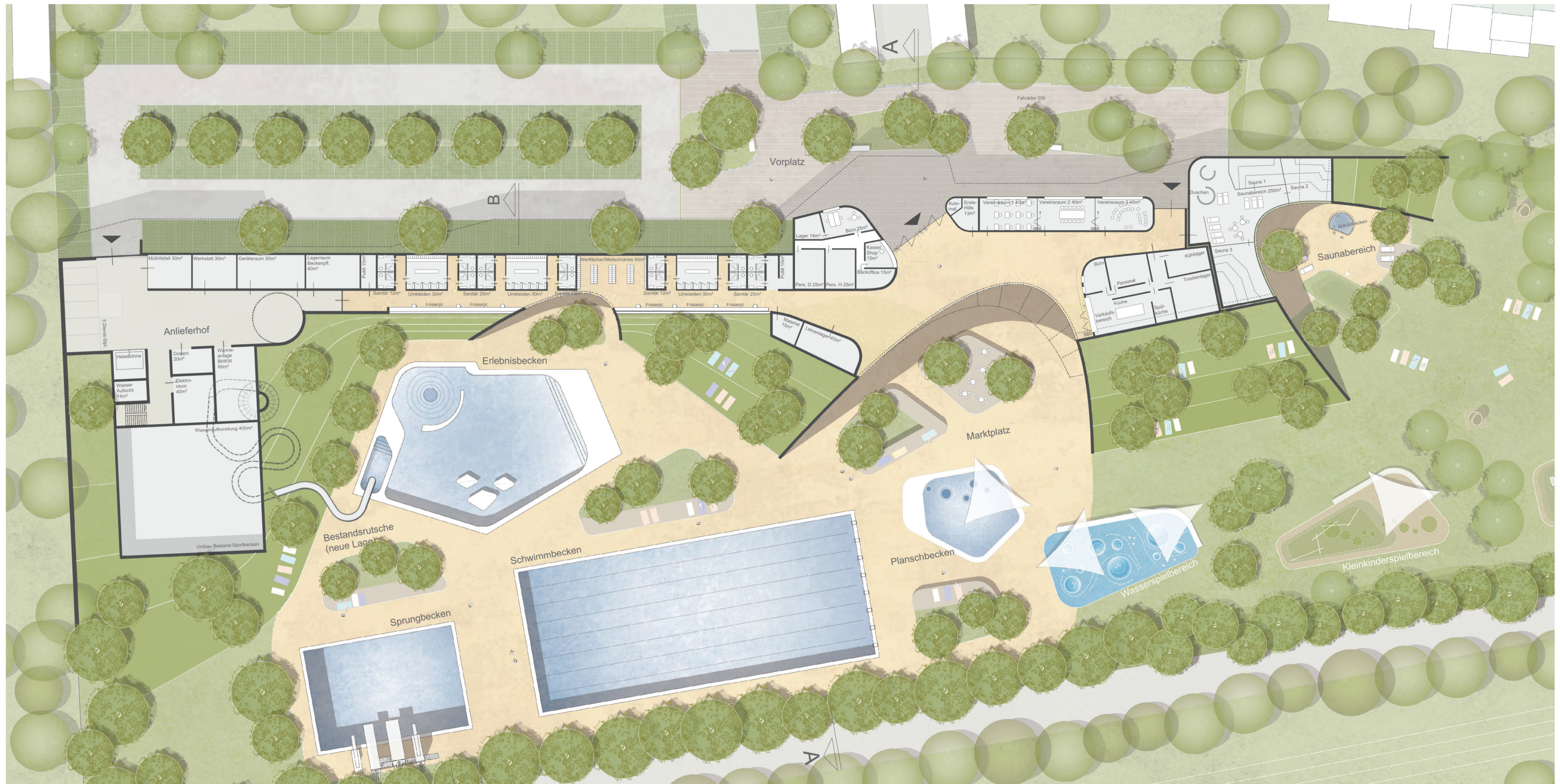
GRUNDRISS EG | 1:200
